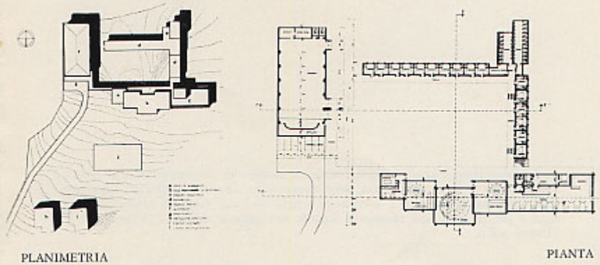
PLANIMETRIA
